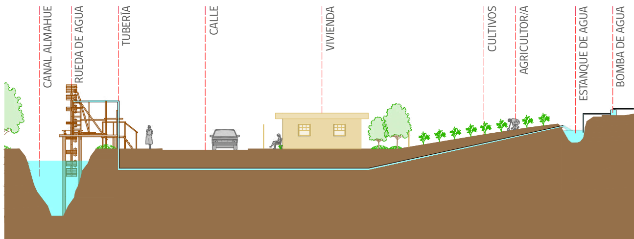
Figura 2: Esquema del sistema de regadío
